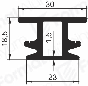
Pr.No: 9363 0,514 kg/m
