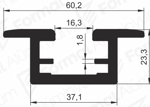
Pr.No: 9404 1,190 kg/m
