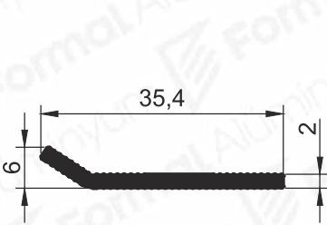
Pr.No: 9770 0,185 kg/m
