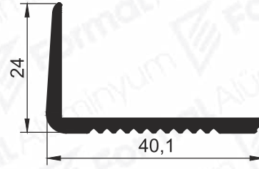
Pr.No: 9147 0,336 kg/m
