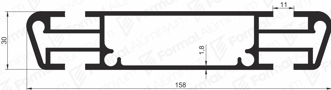
Pr.No: 9315 2,8 kg/m
