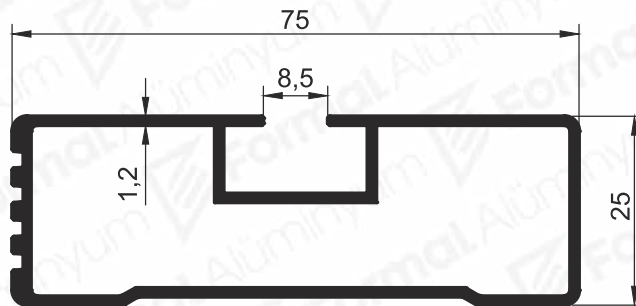
Pr.No: 9840 0,773 kg/m
