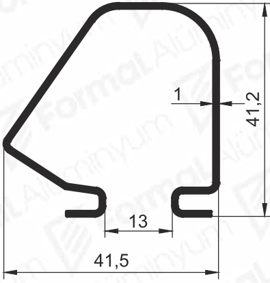
Pr.No: 9917 0,365 kg/m
