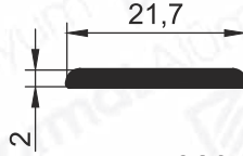
Pr.No: 9231 0,115 kg/m
