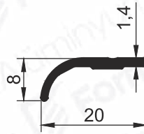
Pr.No: 9347 0,088 kg/m
