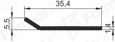
Pr.No: 9124 0,127 kg/m
