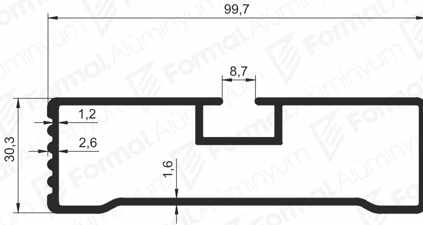
Pr.No: 8732 1,271 kg/m
