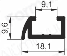
Pr.No: 8946 0,148 kg/m
