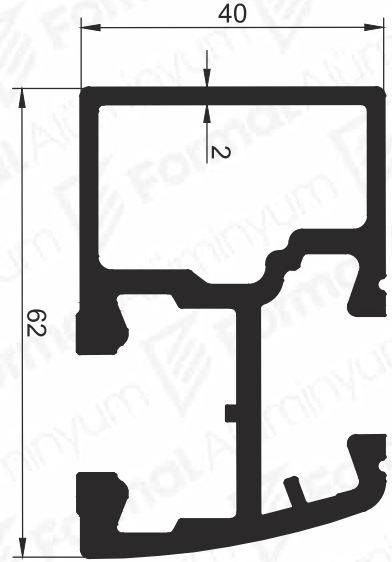
Pr.No: 9314 1,22 kg/m
