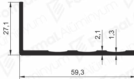
Pr.No: 9194 0,372 kg/m
