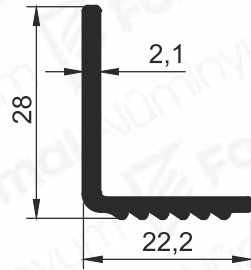
Pr.No: 9233 0,266 kg/m
