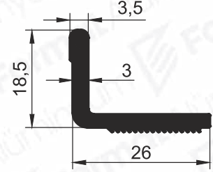
Pr.No: 9000 0,334 kg/m
