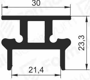
Pr.No: 9313 0,585 kg/m
