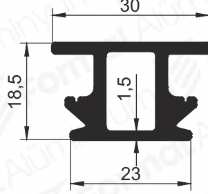
Pr.No: 9362 0,542 kg/m
