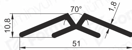
Pr.No: 9448 0,385 kg/m
