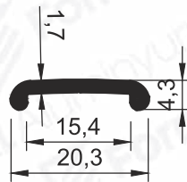
Pr.No: 9197 0,112 kg/m
