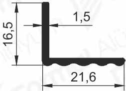
Pr.No: 9232 0,139 kg/m
