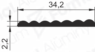
Pr.No: 9230 0,184 kg/m
