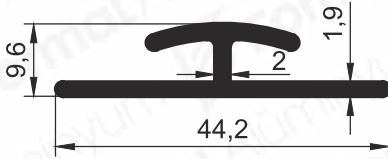
Pr.No: 9196 0,366 kg/m
