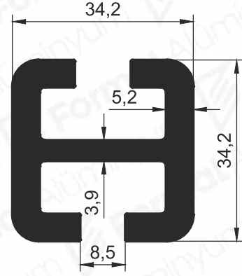
Pr.No: 9325 1,554 kg/m
