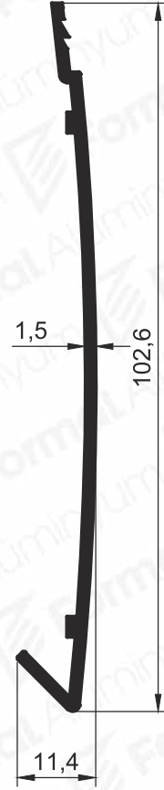
Pr.No: 1034 0,481 kg/m
