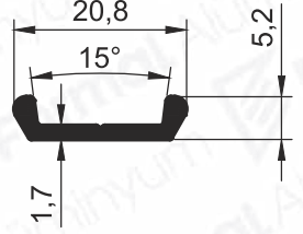
Pr.No: 1267 0,124 kg/m
