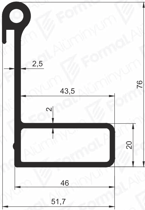
Pr.No: 1030 1,281 kg/m
