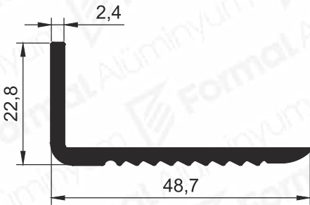
Pr.No: 9378 0,453 kg/m
