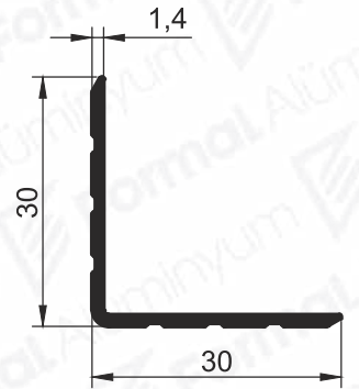
Pr.No: 9147 0,336 kg/m
