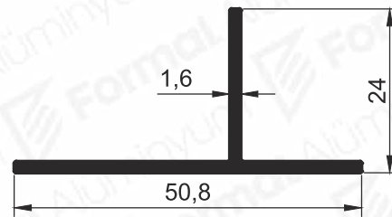
Pr.No: 2616 0,324 kg/m
