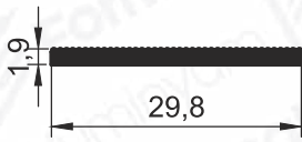
Pr.No: 9146 0,133 kg/m
