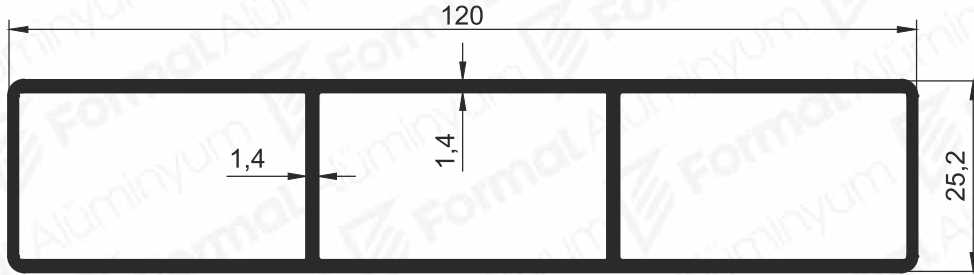
Pr.No: 8972 1,206 kg/m
